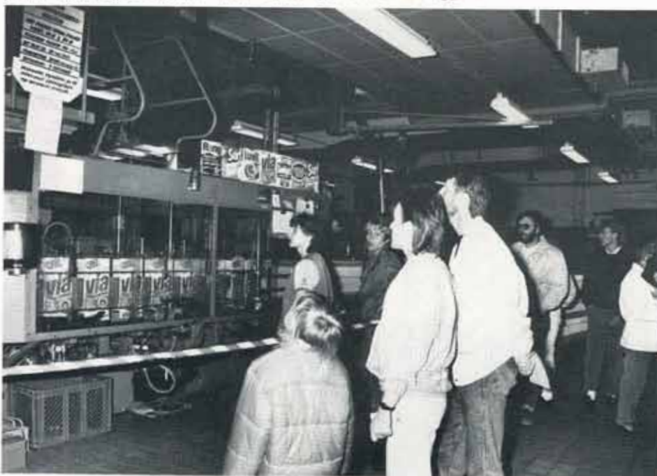
ACMA PULVERPACKNINGSMASKIN packar stora paket med en hastighet av 100/min. Det blir ca 80 ton/skift. - Klarar vi frågan vilka länder Lever tillverkar produkter åt förutom Sverige?
